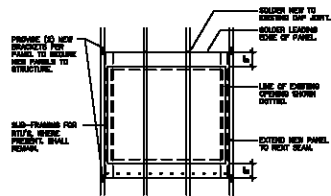
PLAN SCALE: 1/4" = 1'-0"
