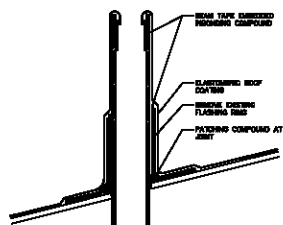
7 VENT FLASHING A103 SCALE: 1 1/2" = 1'-0"
