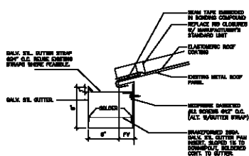
9 CUTTER A103 SCALE: 1 1/2" = 1'-0"
