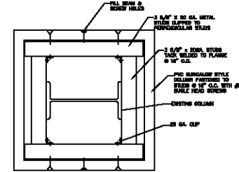
2 COLUMN ENCLOSURE (A31) SCALE: 3" = 1'-0"
