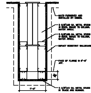
1 COLUMN ENCLOSURE (A31) SCALE: 1 1/2" = 1'-0"
