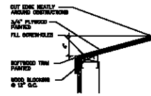
3 WALL CAP (A31) SCALE: 1 1/2" = 1'-0"
