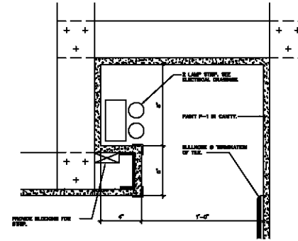
2 LIGHT COVE (A31) SCALE: 3" = 1'-0"
